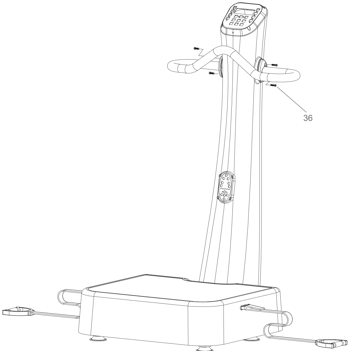
Teil 36 - Schraube M8x25 Menge: 4 Stück
